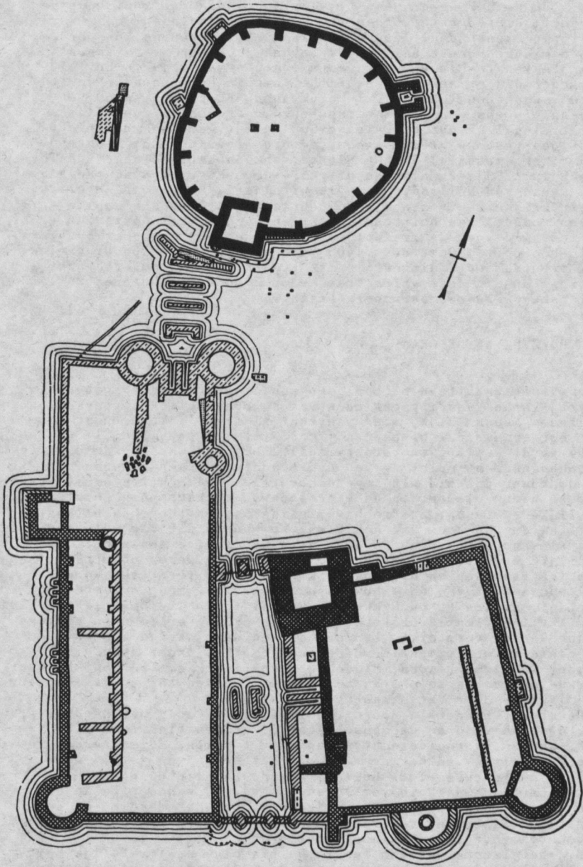
Plattegrond van Egmond zoals het in de loop van de 13e eeuw tot en met de 16e eeuw werd gebouwd.
