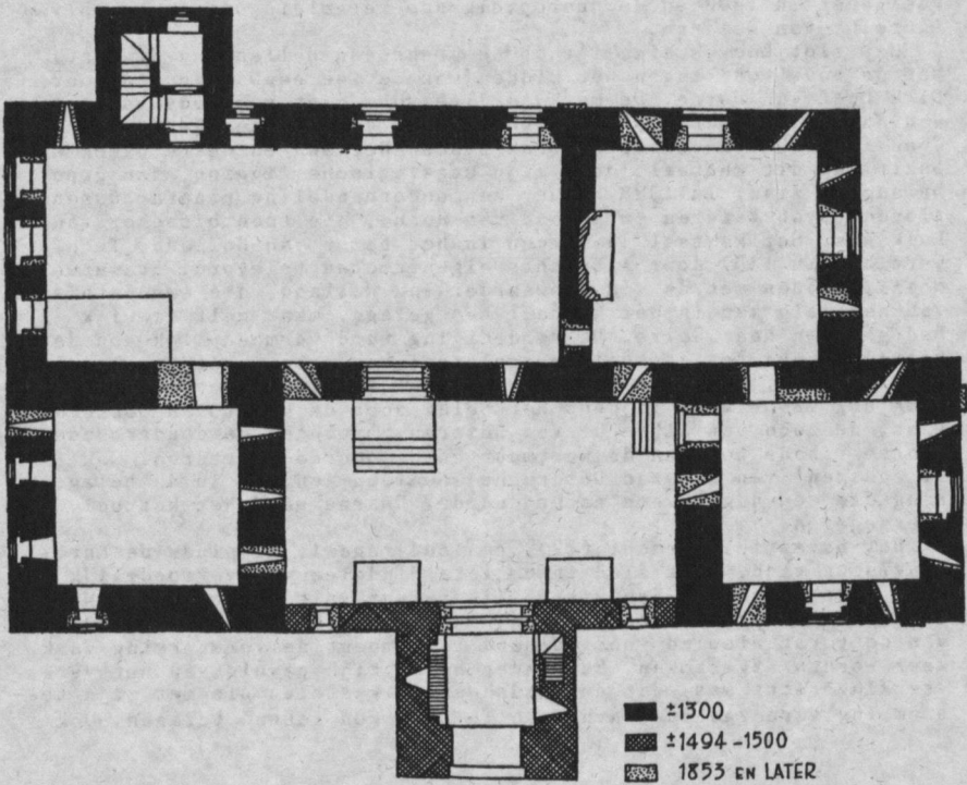
Plattegrond van de kelderverdieping van Loevestein
