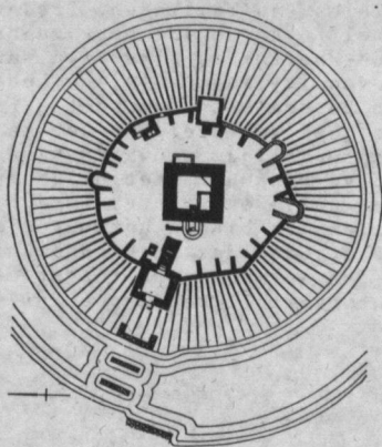
Plattegrond van de burchtheuvel van Oostvoorne
