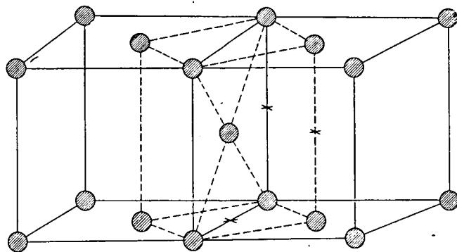
Fig. 10. De vlakkegecentreerd kubische structuur opgevat als tetragonaal ruimtelijk gecentreerd rooster (zie prisma in het midden). Duidelijkheidshalve zijn niet alle Fe-atomen ingetekend. Met kruisjes zijn enkele plaatsen voor interstitiële atomen aangeduid. Deze bevinden zich in de middens van de kubussen en van de ribben van het vlakkegecentreerde rooster.
