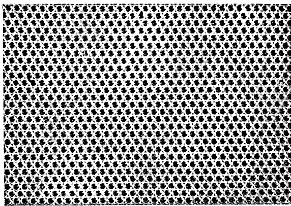
Fig. 3. Een dichtst gepakte laag zeepbelletjes ( Bragg en Nye 20 ). Zie ook fig. 4a. De kristalstructuren in fig. 1b en 1c worden verkregen door deze lagen zo op elkaar te stapelen dat de bolletjes in de kuultjes van de laag er onder komen. In de hexagonale pakking (fig. 1c) zijn de projecties van 1e, 3e, 5e . . . . laag identiek. In de kubische pakking is dat met de 1e, 4e, 7e . . . . laag het geval: ze liggen hier langs (111) vlakken (zie fig. 1b).
