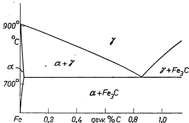
Fig. 6. Deel van het systeem Fe—C beneden 1000° C. Het cementiet (Fe 3 C) zelf, met 6,7 % C, valt buiten de figuur.
