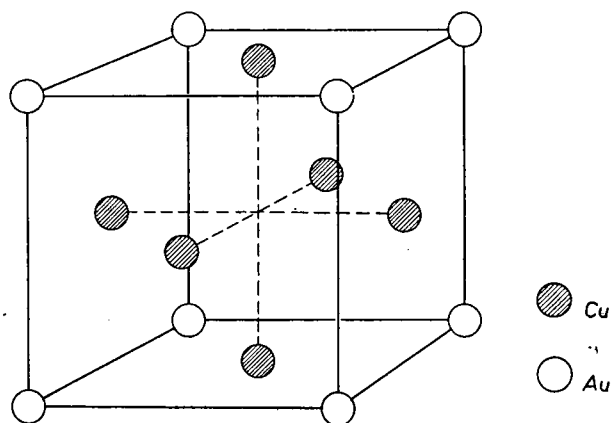
Fig. 8. De superstructuur van Cu 3 Au. In de superstructuur CuAu zijn de middens van boven- en ondervlak van de elementaircel door Au i.p.v. Cu ingenomen. De (100) vlakken zijn dan afwisselend met Cu- en Au-atomen bezet, hetgeen ten gevolge heeft dat die structuur tetragonaal is.
