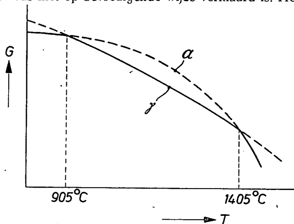
Fig. 2. Schematisch verloop van de vrije enthalpie van de beide modificaties van Fe als functie van de temperatuur.
