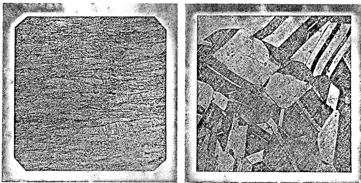
Fig. 5. Rekristallisatie van messing met 20% Zn. Links: koud gewalst. Rechts: daarna gegloeid. De preparaten zijn na polijsten geëët met \text{FeCl}_3 + \text{HCl} . Vergroting 350 \times (Ontleend aan P. Goerens , Einführung in die Metallographie, Halle 1932).
