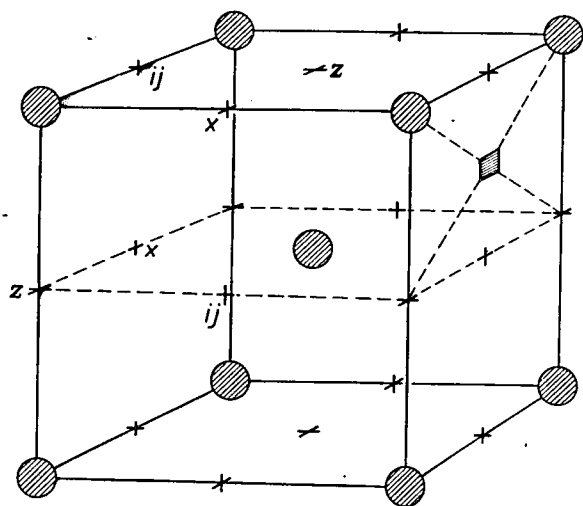
Fig. 9. In \alpha -Fe zitten de C- (of N-)atomen waarschijnlijk niet op de door een vierkantje aangeduide soort plaatsen, maar op (een kleine fractie van) de met kruisjes aangeduide. Middens van de vlakken en van de ribben zijn identiek. De onderscheiding in x-, y- en z-plaatsen is echter van belang.
