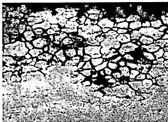
Fig. 11: Interkristallijne corrosie van een Al—Cu legering. Ongeëtste doorsnede van een draad. Vergroting 160 × (Ontleend aan G. Sachs, Praktische Metallkunde III, Berlin, 1935 ).
