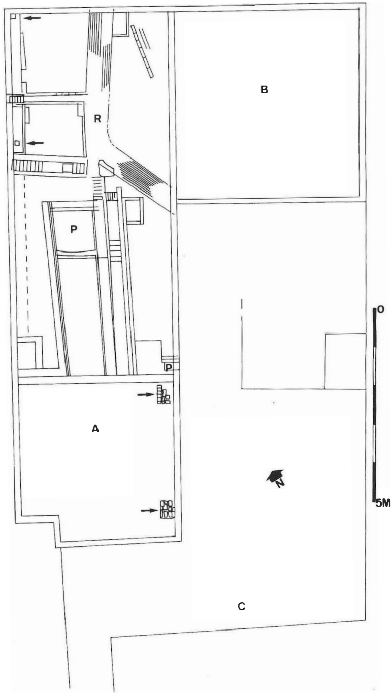
Fig. 1. A = loods, B = keuken, C = binnenplaats, P = put en R = riool. De kleine pijlen geven de standplaatsen aan van de staanderbalken.
