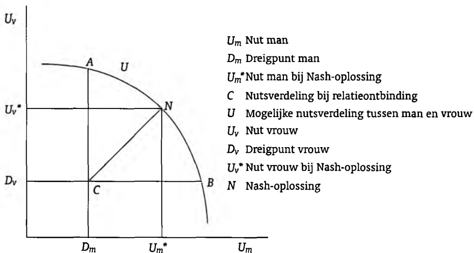
Figuur 1 Onderhandelingsmodel met Nash-oplossing
